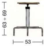
S 30 Sgabello tondello. Round stool.
