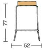
S 2 Sgabello fisso alto. High fixed stool.
