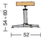
S 14 Sgabello tondello. Round stool.
