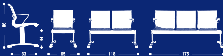
PL15 Sedia fissa con braccioli Fixed armchair
