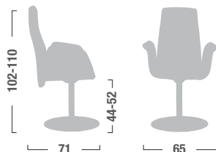
LD15-LDC25-LDW25 Poltrona visitatore con braccioli senza oscillante. Swivelling armchair.
