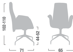
LD14-LDC24-LDW24 Poltrona visitatore con braccioli senza oscillante. Swivelling armchair.
