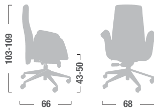
LD13-LDC23-LDW23 Poltrona direzionale con braccioli e oscillante mov. 19. Directional armchair with mov. 19 tilting.
