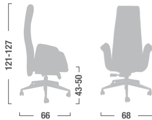
LD11-LDC21-LDW21 Poltrona presidenziale con braccioli e oscillante mov. 19. Presidential armchair with mov. 19 tilting.
