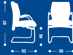
FX38 Poltrona attesa fissa con braccioli. Fixed armchair.
