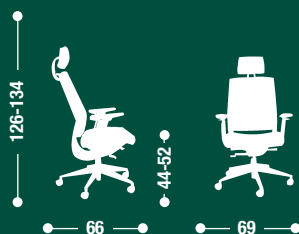
VS 31-VS 41 Poltrona presidenziale con braccioli e oscillante mov. 24 Presidential armchair with mov.24 tilting
