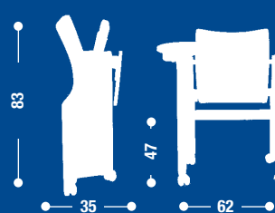
MG33 Pozzetto pieghevole e scrittoio nero. Folding armchair and black writing board.
