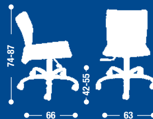
MG35 Sedia girevoli senza braccioli. Swivel chair.
