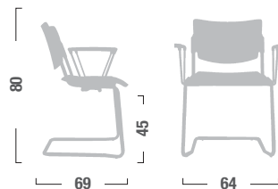
LA22 Sedia fissa a slitta con braccioli. Sledge fixed chair with armrest.
