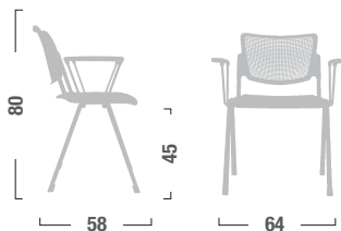
LA12 Sedia fissa a 4 gambe con braccioli. Four legs fixed armchair.
