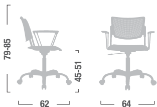
LA16 Sedia girevole con braccioli. Revolving chair with armrests.
