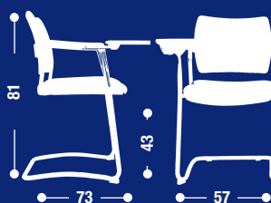
DR25 Sedia fissa con un bracciolo e scrittoio. Fixed chair with armrest and writing board.
