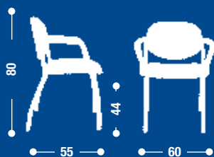
BK6 Sedia fissa con braccioli. Fixed armchair.
